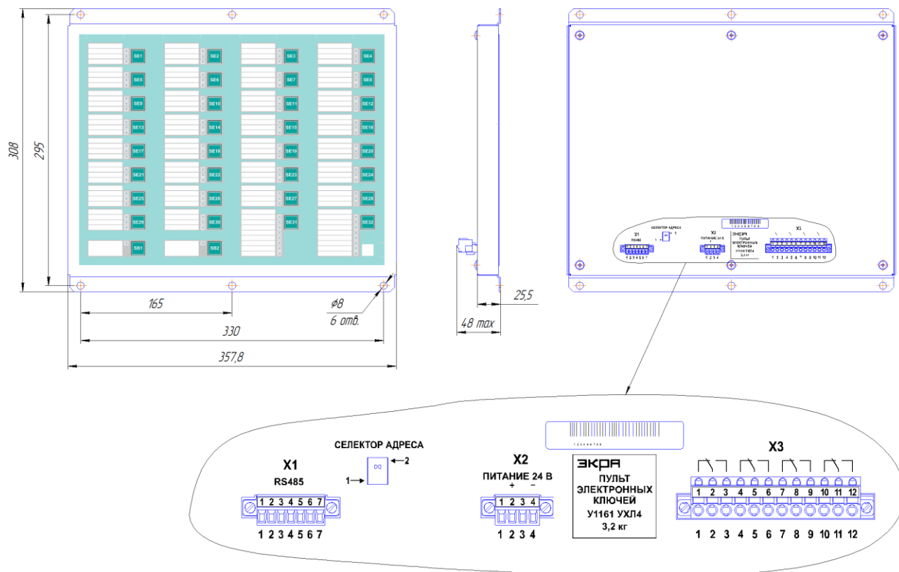
Рисунок 1 – Общий вид и габаритные размеры пульта электронных ключей У1161
